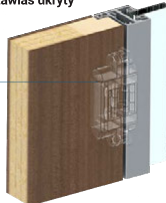
Zawias ukryty
